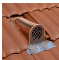
Haube NE Kupfer Großflächenziegel
